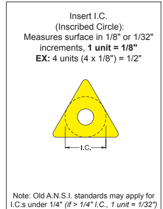
9. Insert Size I.C.
