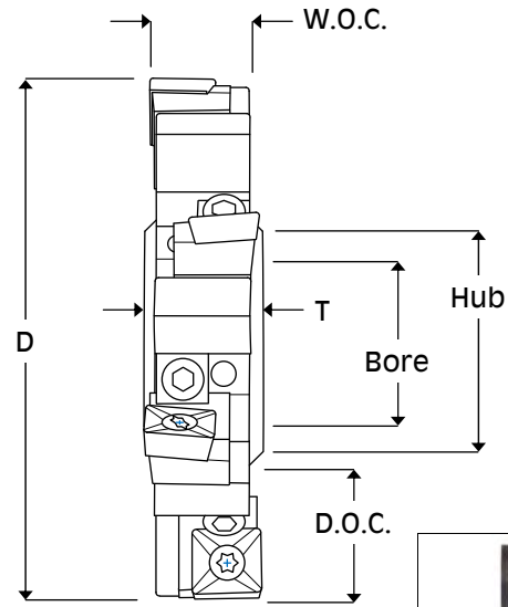
R.H. Cartridge
