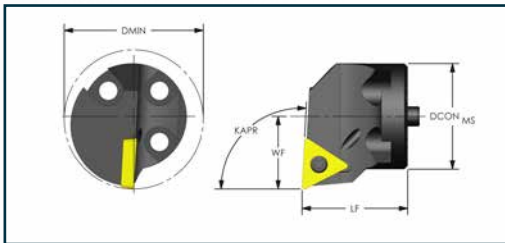
Positive Triangle (KAPR:93°)
