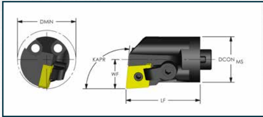
Negative 80° Diamond (KAPR: 95°)
