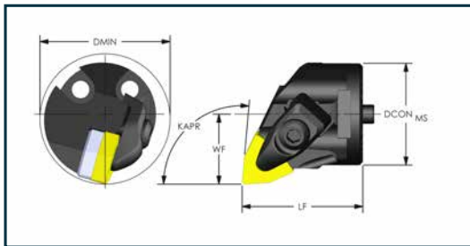
PULLBACK Clamp Negative Trigon (KAPR: 95°)
