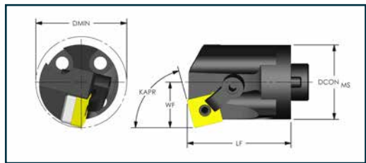
Negative Square (KAPR: 75°)
