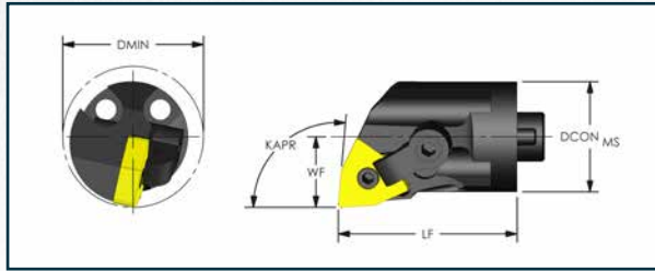
Negative Trigon ( KAPR: 95°)
