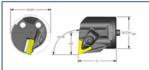
PULLBACK Clamp Negative Triangle (KAPR: 93°)
