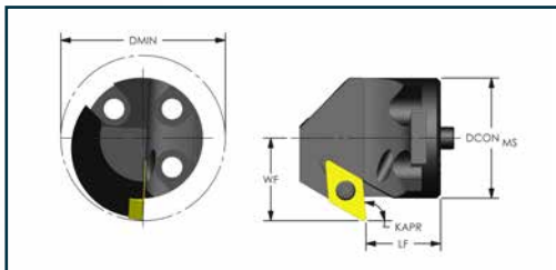
Positive 55° Diamond (KAPR: 95°) Back Facing
