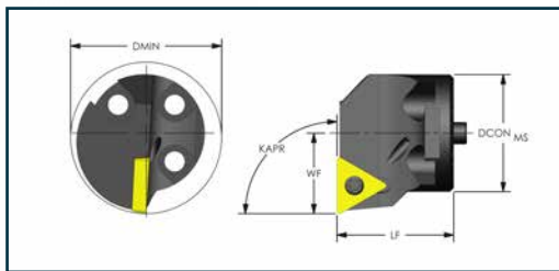
Positive Triangle (KAPR:90°)
