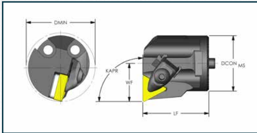
PULLBACK Clamp Negative Triangle (KAPR: 90°)
