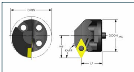
Positive 55° Diamond (KAPR: 62.5°) Profiling
