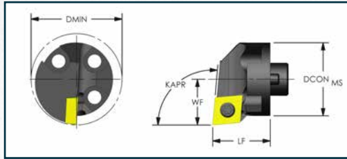
Positive 80° Diamond (KAPR: 93°)
