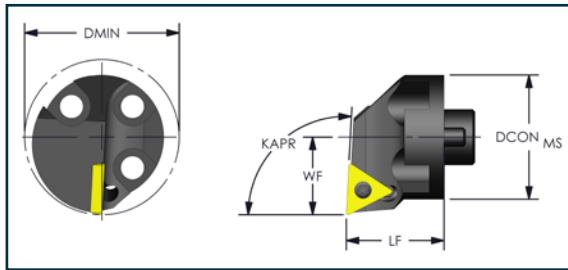
Positive Triangle (KAPR: 93°)
