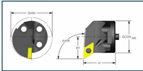
Positive 55° Diamond (KAPR: 93°) Profiling
