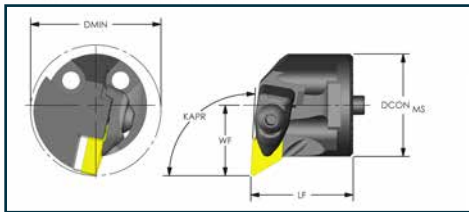
PULLBACK Clamp Negative 55° Diamond (KAPR: 93°)
