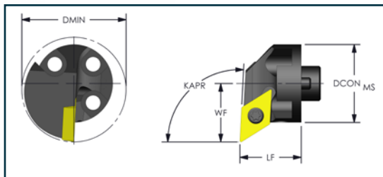
Positive 55° Diamond (KAPR: 93°) Profiling
