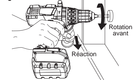
Fig. 7 Étayage contre la jambe
