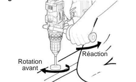
Fig. 8 Étayage contre un montant
