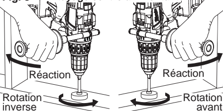
Fig. 8 Étayage contre un montant
